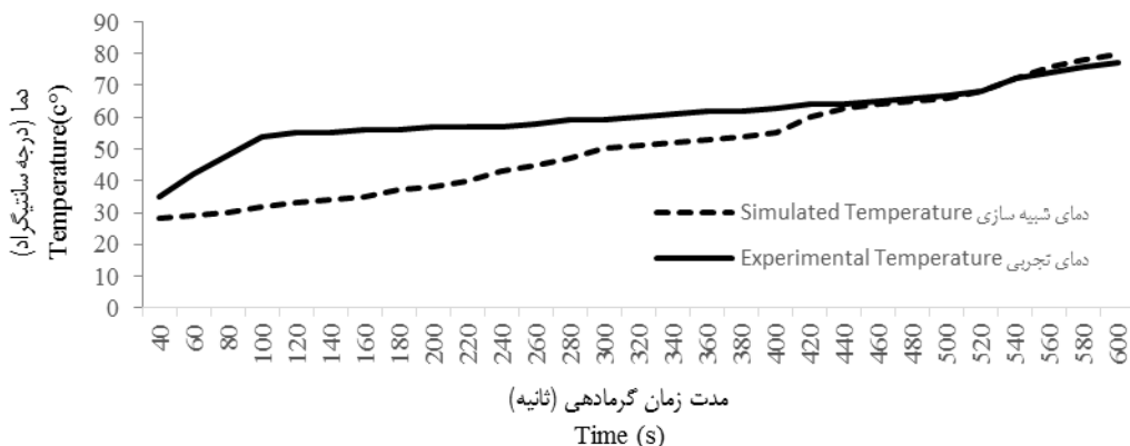
شکل ۹- نمودار دمای شبیه‌سازی شده و دمای تجربی در نقطه ۱ متناسب با مدت گرمادهی
