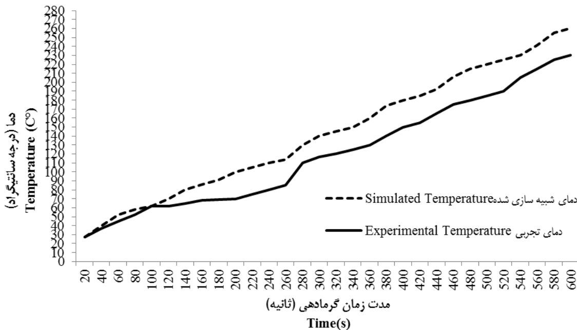
شکل ۱۰- نمودار دمای شبیه‌سازی شده و دمای تجربی در نقطه ۲ متناسب با مدت گرمادهی
