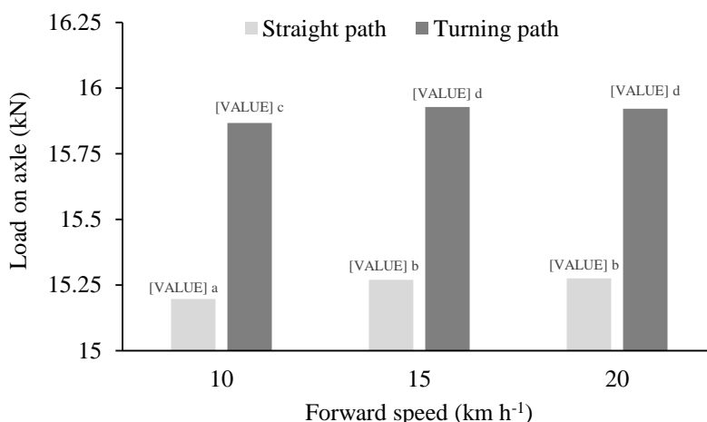
شکل ۷- میانگین بارهای عمودی وارده بر اکسل عقب کمباین در جاده آسفالت
