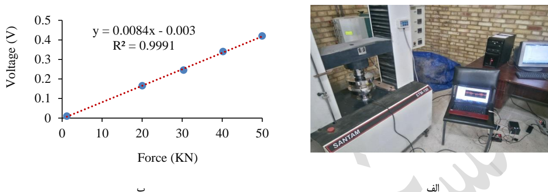
شکل ۴- الف) نحوه باردهی به نیروسنج در دستگاه آزمون کشش- فشار و ب) نمودار کالیبراسیون نیروسنج Fig. 4. a) Loading method of loadcell in a universal testing machine and b) Loadcell calibration curve
