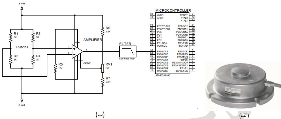
شکل ۲- الف) نیروسنج دیسکی فشاری و ب) مدار تقویت کننده و فیلترکننده ولتاژ خروجی نیروسنج Fig. 2. a) Disc type compression loadcell and b) Amplifier and filter circuit for the loadcell output voltage
