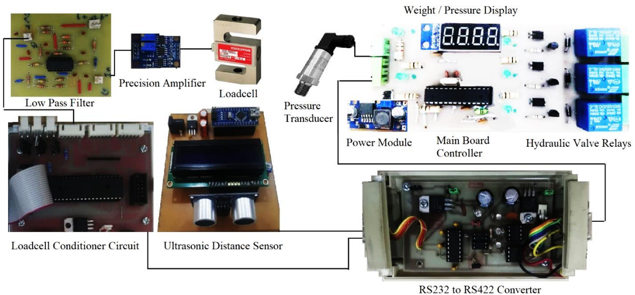
شکل ۶- اجزای سخت‌افزاری سامانه کنترل خودکار (مدارهای کنترل، حسگرهای وزن، فراصوت و فشار) و نحوه ارتباط آن‌ها Fig.6. Automatic control system parts (control, weight, ultrasonic, and pressure circuit) and their connections
