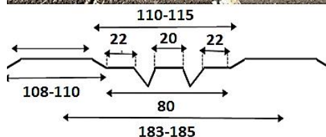
شکل ۷- ابعاد جوی و پشته (سانتی‌متر) و نحوه اندازه‌گیری مصرف وزنی ریزش قلمه و فواصل نداشت
