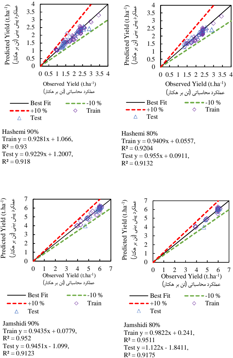
شکل 4- پراکندگی مقادیر محاسباتی در برابر مقادیر پیش‌بینی شده عملکرد شلتوک Fig.4. Cross correlation of the observed and predicted values of paddy yield
