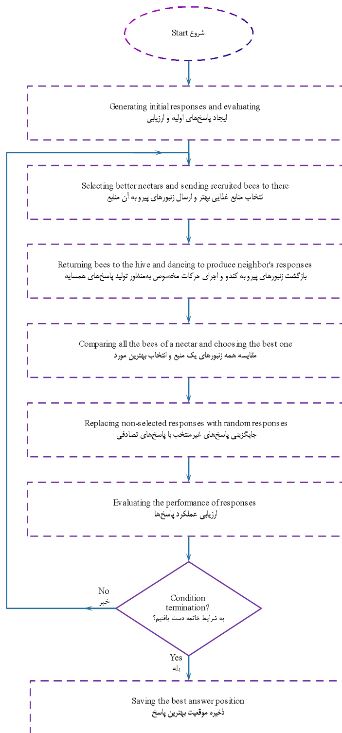
شکل 2- الگوریتم زنبور عسل مصنوعی Fig.2. Artificial Bee Colony algorithm
