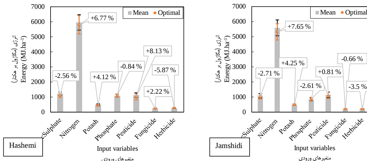
شکل 7- مقایسه مقادیر انرژی مصرفی و بهینه متغیرهای ورودی (خطوط مشکی و قرمز به ترتیب نشانگر انحراف معیار مقدار میانگین و بهینه می‌باشند)
