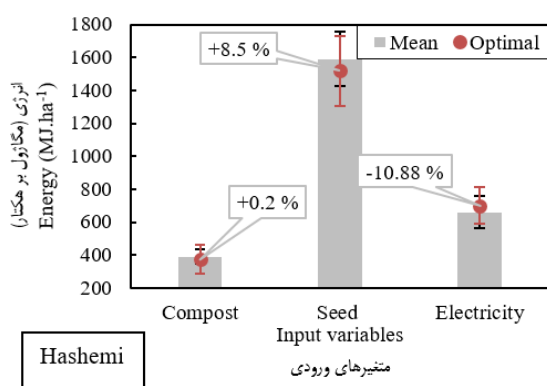
شکل 6- مقایسه مقادیر انرژی مصرفی و بهینه متغیرهای ورودی (خطوط مشکی و قرمز به ترتیب نشانگر انحراف معیار مقدار میانگین و بهینه می‌باشند)
