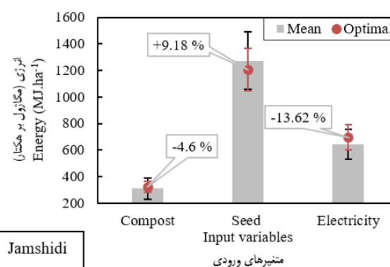
شکل 6- مقایسه مقادیر انرژی مصرفی و بهینه متغیرهای ورودی (خطوط مشکی و قرمز به ترتیب نشانگر انحراف معیار مقدار میانگین و بهینه می‌باشند)
