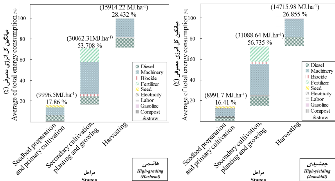
شکل 3- سهم توزیع انرژی ورودی‌ها در سه مرحله (مگاژول بر هکتار) Fig.3. Share of energy input distribution across three stages (MJ.ha -1 )
