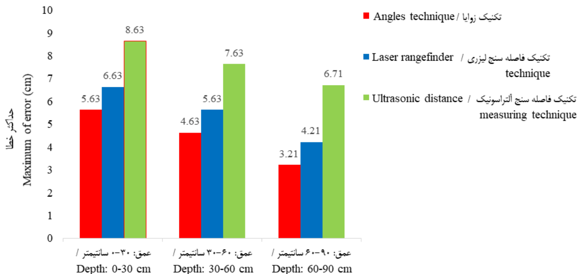
شکل ۹- مقایسه حداکثر خطاهای عمق مربوط به اثر متقابل روش‌های مختلف عمق‌سنجی و دامنه‌های متفاوت عمق
