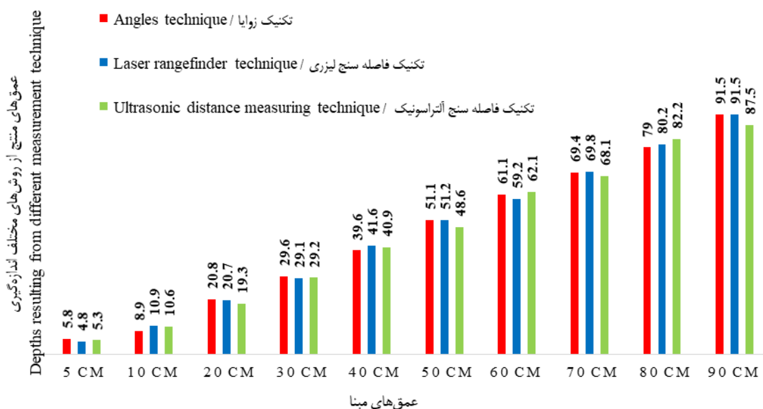
شکل ۵- صحت‌سنجی سامانه بر روی سکوی ثابت Fig.5. System calibration on a fixed platform
