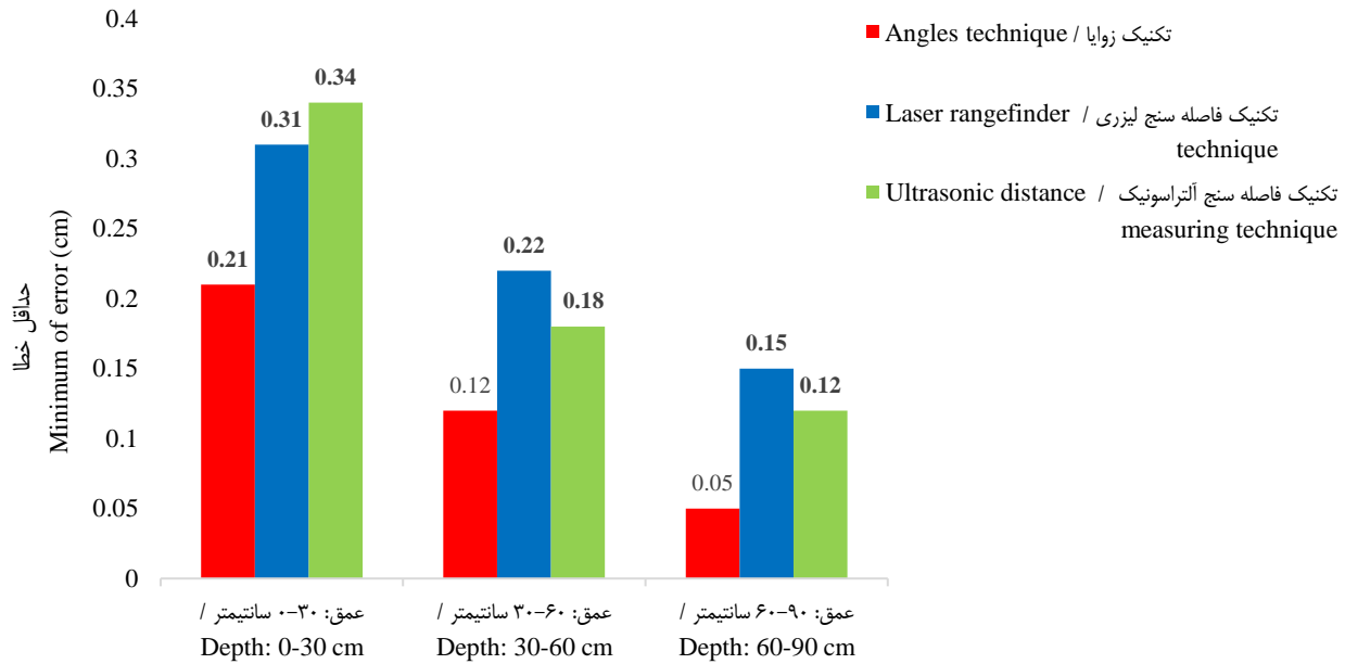
شکل ۸- مقایسه حداقل خطاهای عمق مربوط به اثر متقابل روش‌های مختلف عمق‌سنجی و دامنه‌های متفاوت عمق
