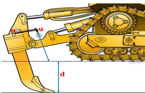
ب- سنجش عمق ( d ) با استفاده از فاصله سنجی به وسیله حسگر فراصوتی ( u ) و زاویه متغیر این حسگر نسبت به افق ( \alpha )
