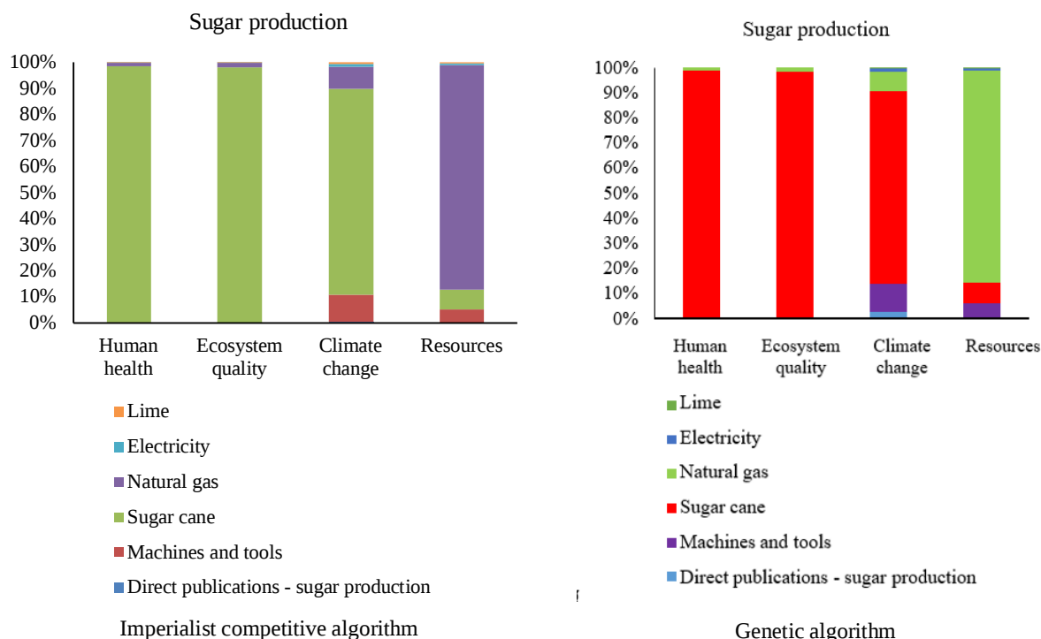
شکل 1- سهم هر یک از نهاده‌های مصرفی و تأثیر آن‌ها در دسته خسارات در کارخانه تولید شکر پس از بهینه‌سازی Fig.1. The contribution of each of the consumption inputs and their effect in the category of damages in the sugar factory after optimization
