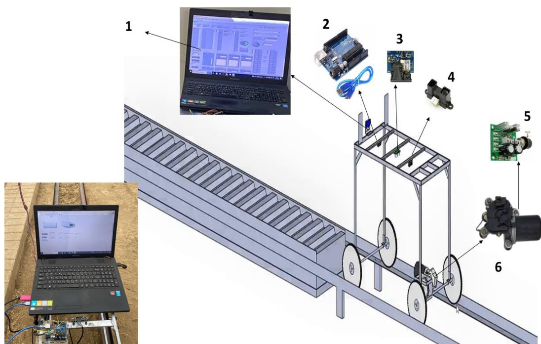
شكل ۵- طرح‌واره سامانه درحال حرکت براي اندازه‌گيري زبري بلادرنگ خاك: ۱) لپ‌تاب، ۲) برد آردوينو، ۳) حسگر ليزر، ۴) حسگر مادون قرمز، ۵) كنترلر دور الكتروموتور و ۶) الكتروموتور
