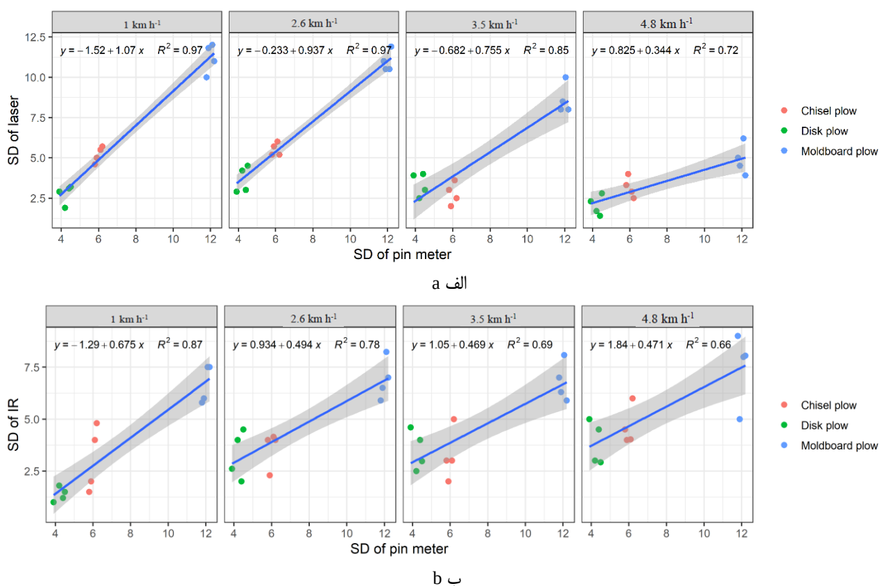
شکل ۱۱- برازش بین زبری اندازه‌گیری‌شده توسط پین‌متر: الف) لیزر و ب) حسگر مادون در سرعت‌های مختلف رو به جلو
