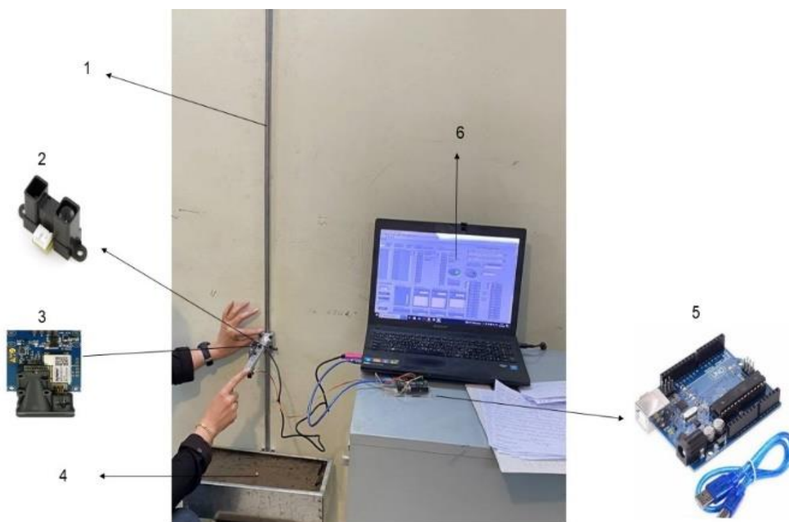
شکل ۲- سامانه واسنجی حسگرها: ۱) ریل هادی، ۲) حسگر مادون قرمز، ۳) حسگر لیزر، ۴) سطح خاک، ۵) برد آردوینو و ۶) لپ‌تاب و نرم‌افزار لپ وینو
