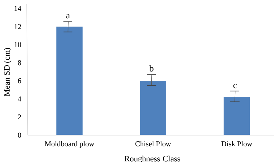
شکل ۹- مقایسه میانگین شاخص زبری تصادفی در کلاس‌های مختلف زبری در آزمایش‌های مزرعه Fig.9. Mean comparison of random roughness index in different roughness classes in field experiments
