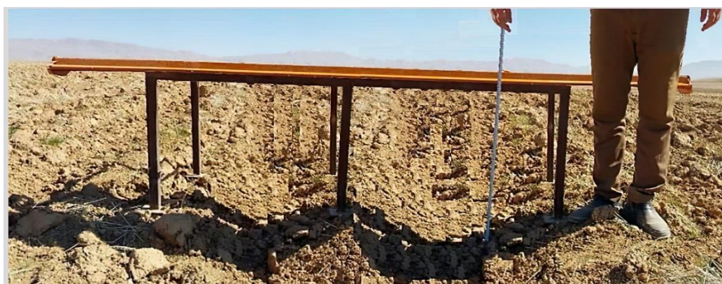
شکل ۱- اندازه‌گیری ناهمواری سطح خاک با استفاده از دستگاه پین متر ساخته شده
