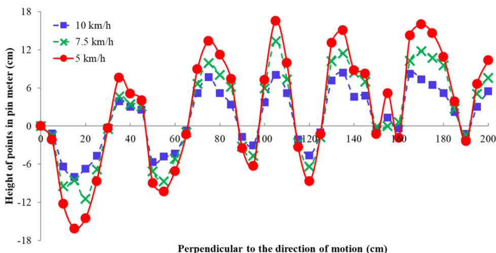
شکل ۵- منحنی‌های پروفیل خاک پس از شخم در سرعت‌های مختلف (عمق ۱۷/۵ سانتی‌متر) Fig.5. Soil profile curves after tillage at various speeds (17.5 cm depth)
