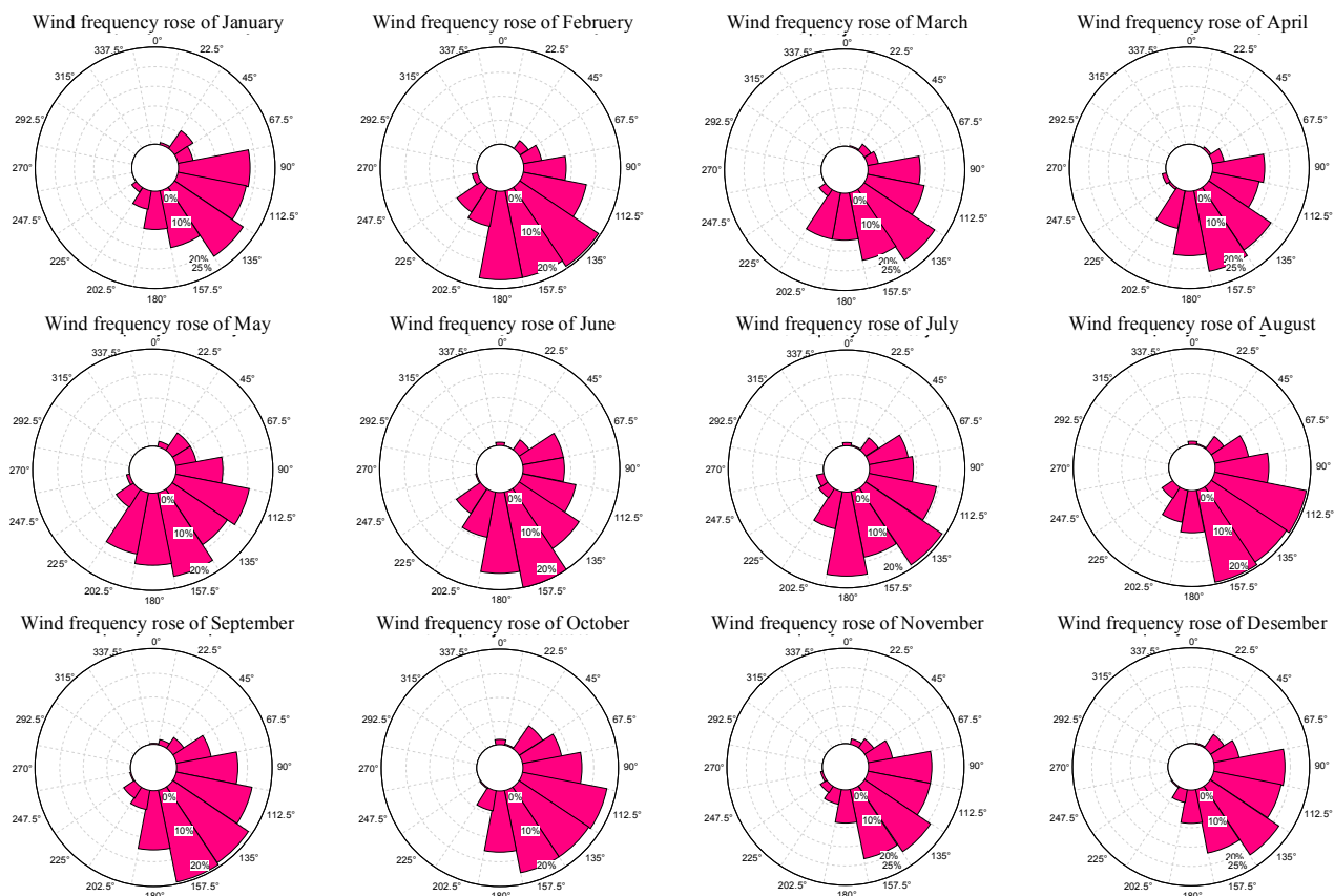
شکل ۱- گلباد جهت باد Fig.1. Wind frequency rose
