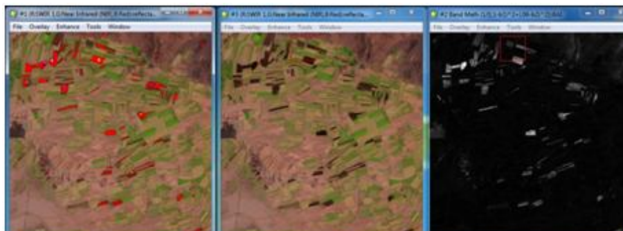
شکل 2- نمونه‌ای از تصویر سنجنده لندست 8 از مزارع آزمایشی (تصویر میانی)، تصویر حاصل از شاخص BAI (تصویر سمت راست) و جداسازی مزارع سوخته با استفاده از آستانه بالا و پایین شاخص BAI (تصویر سمت چپ)
