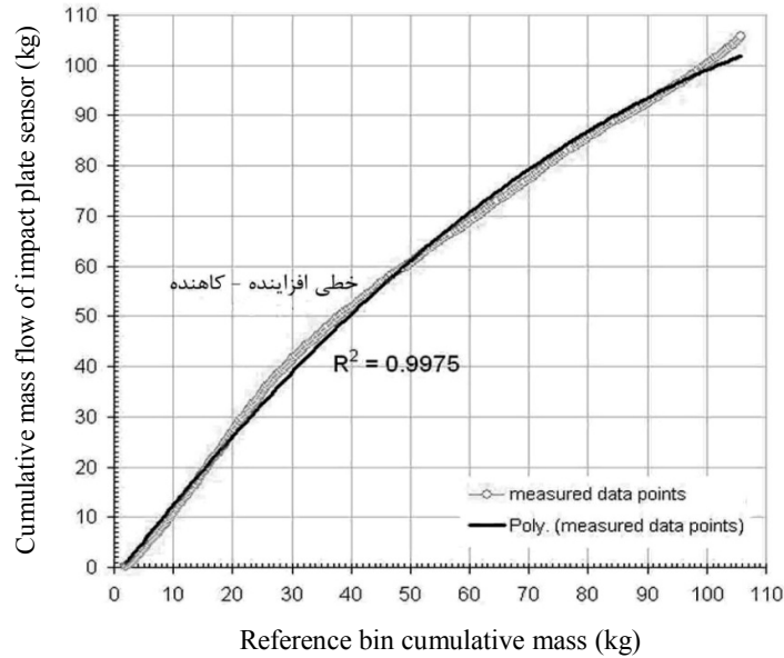
شکل ۱۱- رابطه بین داده‌های تجمعی حسگر ضربه‌ای و بارسنج مخزن مرجع در نرخ جریان جرمی غیر یکنواخت با تغییرات خطی افزایشده-کاهشده
