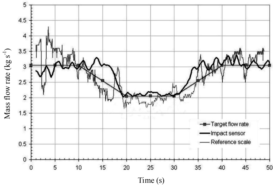
شکل ۱۲- مقایسه داده‌های نرخ جریان جرمی لحظه‌ای حسگر ضربه‌ای و بارسنج مخزن مرجع درحالت نرخ جریان جرمی غیر یکنواخت با تغییرات خطی افزایشده-کاهشده
