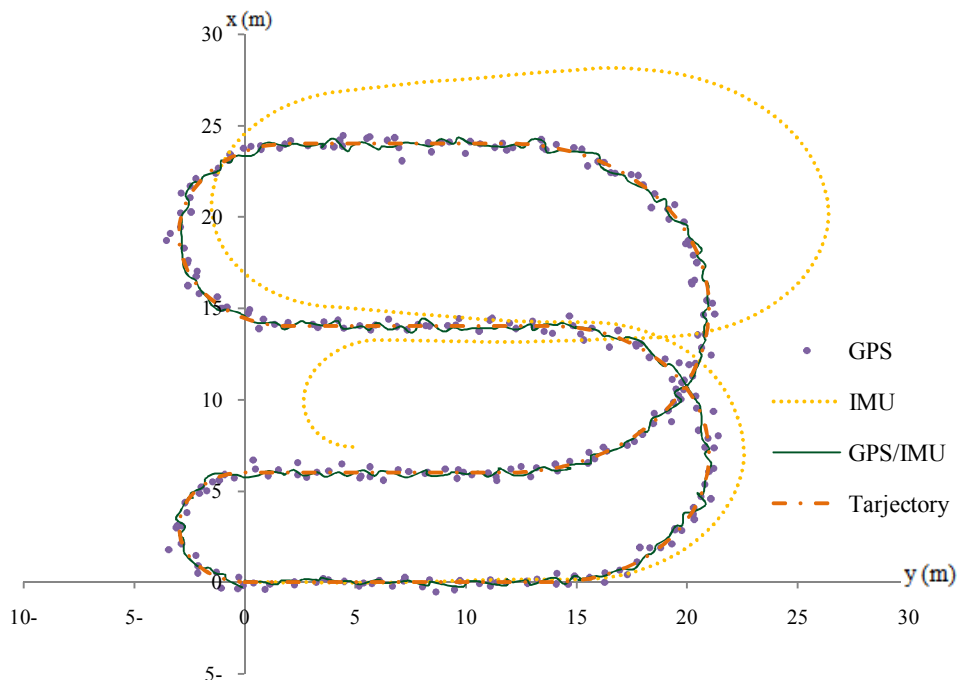
شکل ۱۰- نمایش مسیر حرکت روبات توسط واحد مکان‌یاب جهانی، واحد اندازه‌گیری ماند و تلفیق آن‌ها با یکدیگر Fig.10. Measured robot position using GPS, IMU and GPS/IMU integration
