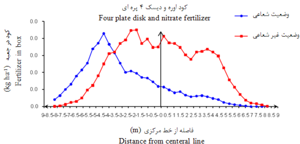
شکل ۴- اثر وضعیت قرارگیری پره بر یکنواختی الگوی پخش کود اوره
