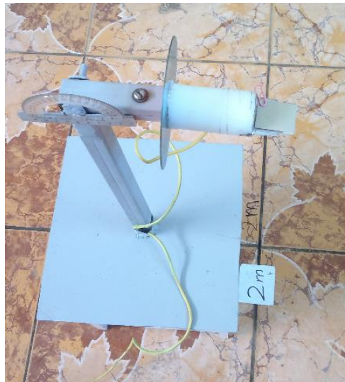
شکل ۲- پایه فلزی متصل به زمین
