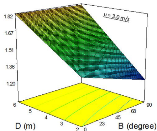
شکل ۵- نمودار سطح پاسخ برای تغییرات ضریب یکنواختی پاشش کل بر حسب پارامترهای مستقل در سرعت هوای ۳ متر بر ثانیه
