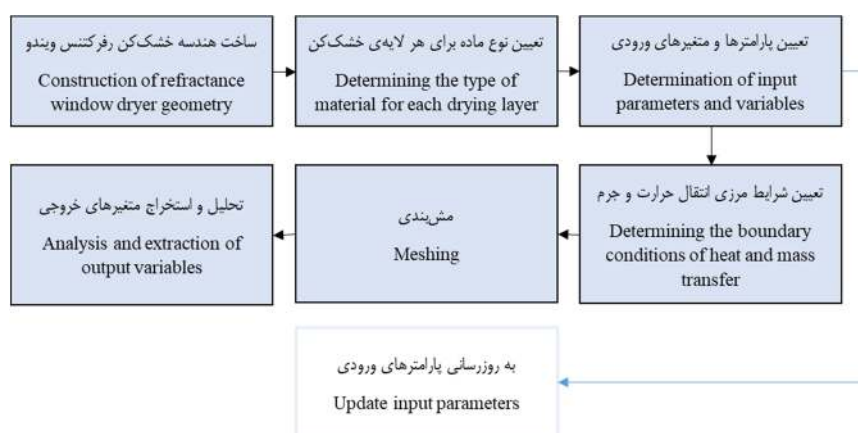
شکل ۱۰- الگوریتم شبیه‌سازی انتقال حرارت و جرم خشک‌کن رفرکتانس ویندو در نرم‌افزار کامسول
