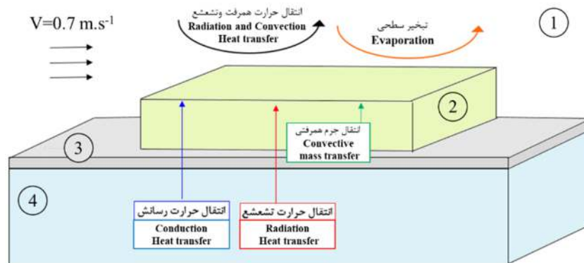
شکل ۳- شماتیک پدیده‌های انتقال در محفظه‌ی خشک‌کن رفرکتانس ویندو (۱- هوا، ۲- ژل آلوئه‌ورا، ۳- فیلم مایلار و ۴- آب)
