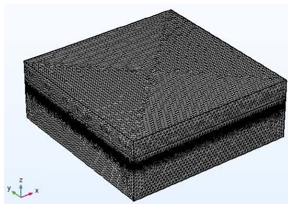
شکل ۹- مش‌بندی نمونه مدل‌سازی شده در نرم‌افزار کامسول Fig.9. Modeled sample meshing in Camsol software
