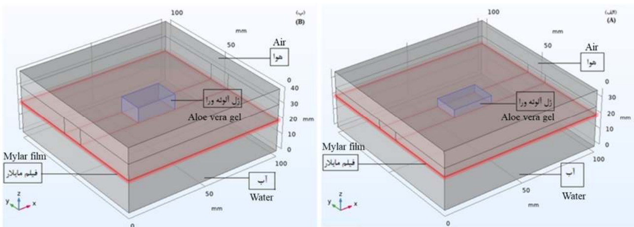
شکل ۲- مدل هندسی ترسیم شده در نرم افزار کامسول با دو ضخامت ژل آلوئه‌ورا: الف) ۵ میلی‌متر و ب) ۱۰ میلی‌متر Fig.2. Geometrical model drawn in Comsol software with two thicknesses of aloe vera gel: A) 5 mm and B) 10 mm
