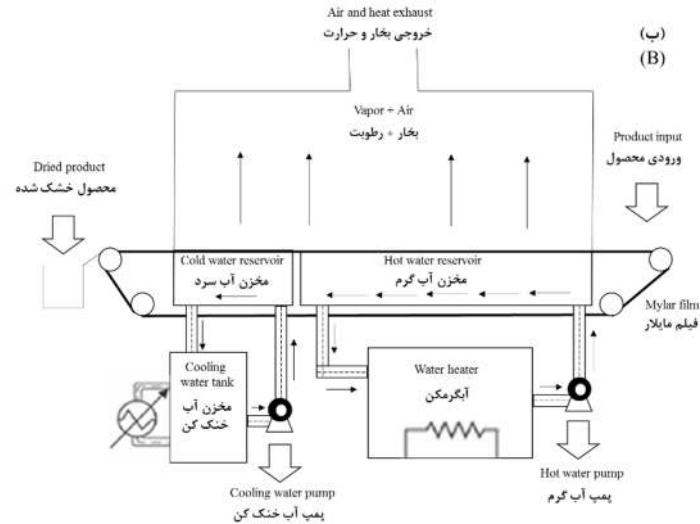
شکل ۱- الف) شکل واقعی خشک کن رفرکتانس ویندو (۱- حمام حرارتی، ۲- مخزن آب، ۳- پمپ آب، ۴- خروجی بخار و حرارت، ۵- فیلم مایلار، ۶- ورودی محصول، ۷- محصول خشک شده و ۸- فن) (واقع در مرکز تحقیقات کشاورزی و منابع طبیعی خراسان رضوی)، ب) شماتیک خشک کن رفرکتانس ویندو و قسمت‌های مختلف آن
