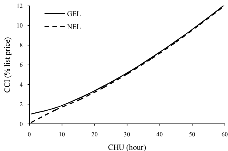
شکل ۵- منحنی GEL و NEL برای کمباین
