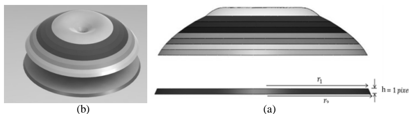
شکل 2- شبیه‌سازی سیب با دوران تمامی المان‌ها a: المان‌بندی سطح تصویر b: دوران المان‌ها
