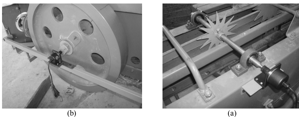
شکل ۳- سامانه‌های اندازه‌گیری؛ (a) ضخامت لایه افزوده در هر مرحله پرس، (b) سرعت خطی پلانجر
