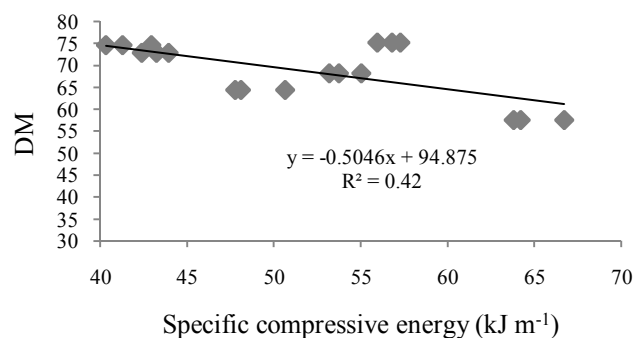
شکل ۹- منحنی واسنجی انرژی فشردگی ویژه و شاخص کیفیت تغذیه‌ای DM Fig.9. Calibration curve for specific compressive energy vs. DM
