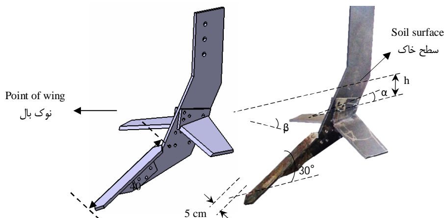
شکل 1- طرحواره و تصویر واقعی ابزار خاک‌ورز قلمی بالدار (h: عمق قرارگیری بال، \alpha : زاویه حمله بال و \beta : زاویه تمایل بال)
