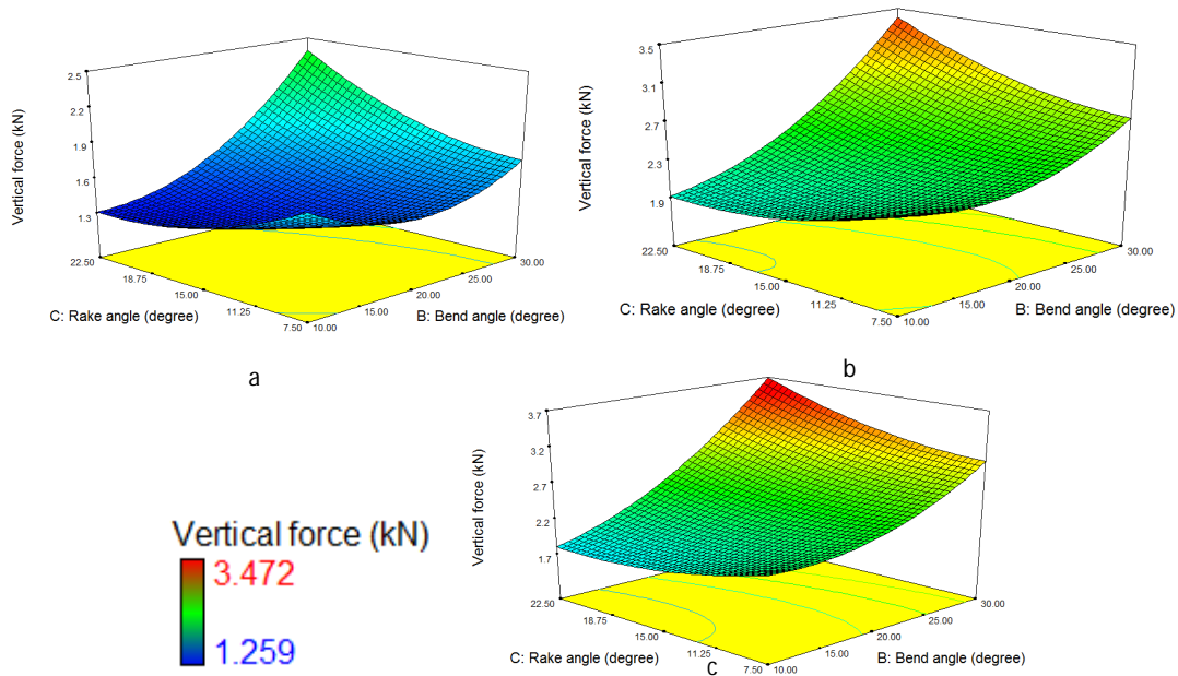
شکل 5- اثرات متقابل زاویه تمایل و حمله بر نیروی عمودی (a: عمق قرارگیری بال = 5 سانتی‌متر، b: عمق قرارگیری بال = 10 سانتی‌متر و c: عمق قرارگیری بال = 15 سانتی‌متر) Fig. 5. The effects of interaction between bend and rake angles on vertical force (depth of wing, a: 5 cm, b: 10 cm, and c: 15 cm)
