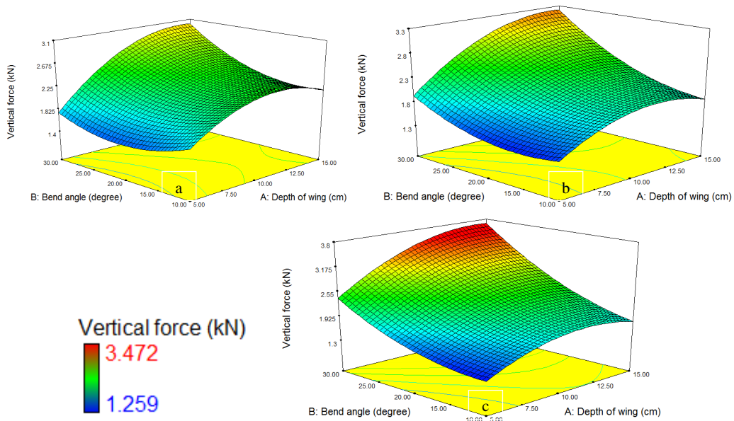
شکل 4- اثرات متقابل عمق قرارگیری و زاویه تمایل بال بر نیروی عمودی (زاویه حمله، a: 7/5 درجه، b: 15 درجه و c: 22/5 درجه) Fig. 4. The effects of interaction between depth of wing and bend angles on vertical force (rake angle, a: 7.5°, b: 10°, and c: 15°)
