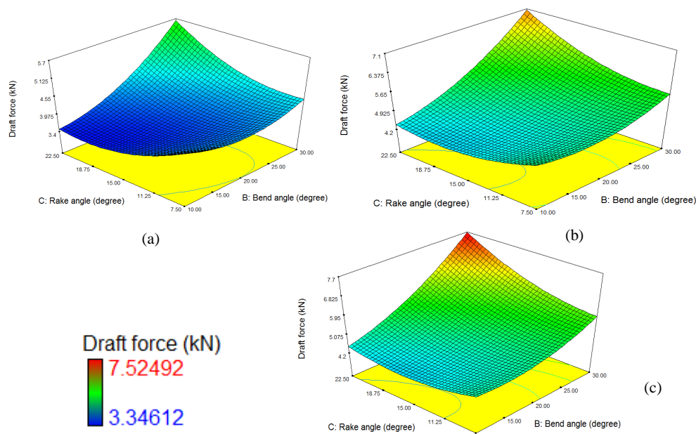
شکل 3- اثرات متقابل زاویه تمایل و حمله بر نیروی کششی (عمق قرارگیری بال، a: 5 سانتی‌متر، b: 10 سانتی‌متر و c: 15 سانتی‌متر) Fig. 3. The effects of interaction between bend and rake angles on draft force (depth of wing, a: 5 cm, b: 10 cm, and c: 15 cm)
